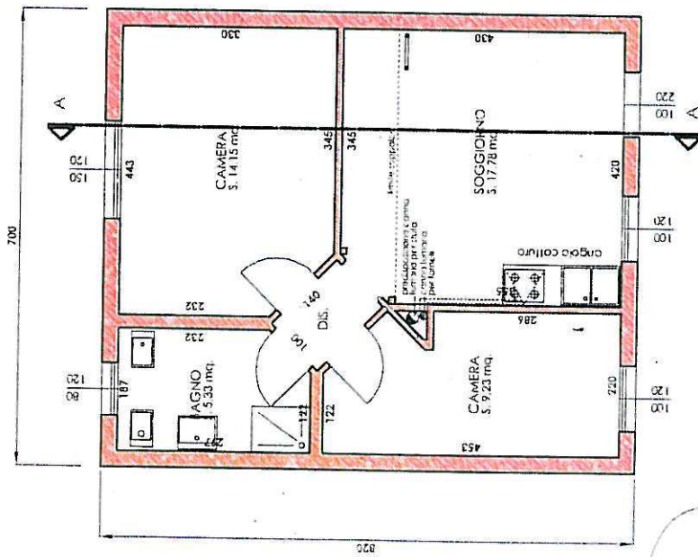
PIANTA UNITA' ABITATIVA scala 1:100
